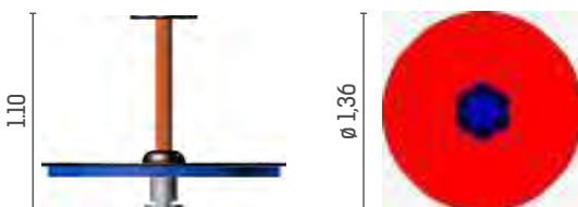
CARRUSEL CON BARANDAS Ref. 81283
